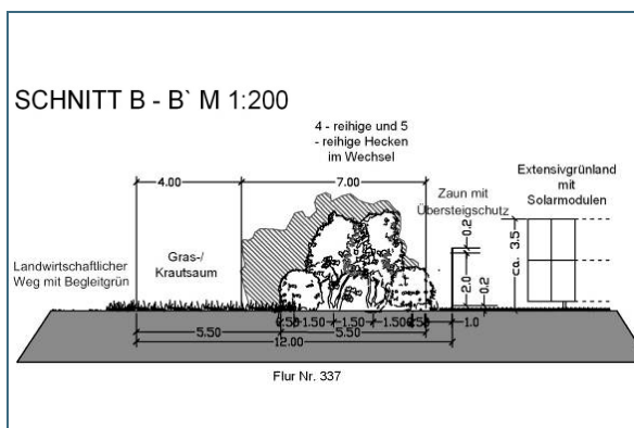
Abb. 56: Querschnitt Grünordnungsplan Plan: J. Ermisch
