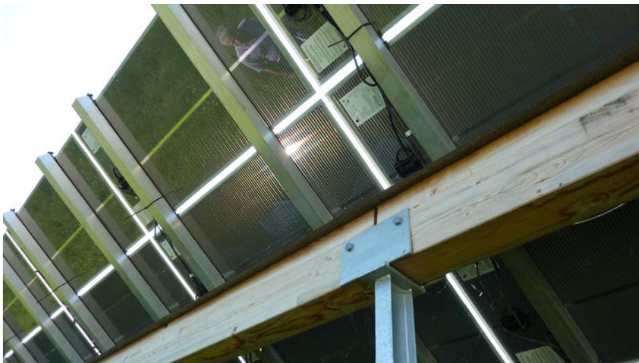
Abb. 26: Wasserablauf zwischen den Modulen durch Abstände
