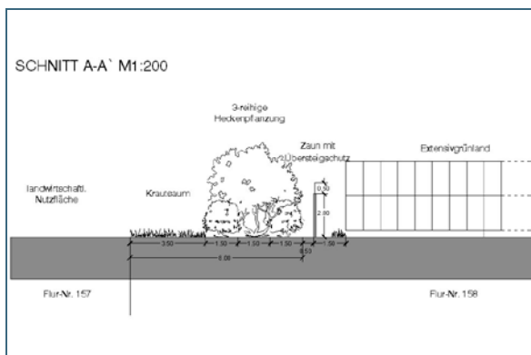
Abb. 53: Heckenpflanzung mit Krautsaum Plan: J. Ermisch
